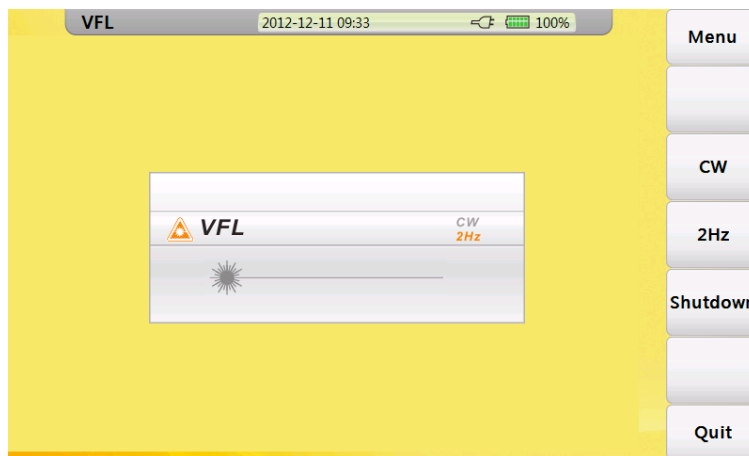
VFL interface
