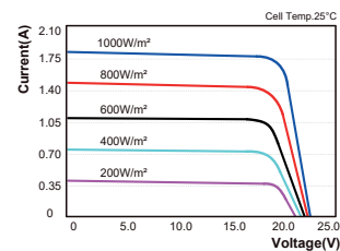
Curvas I-V del módulo PV ESF-30PA I-V Curves of PV module ESF-30PA
