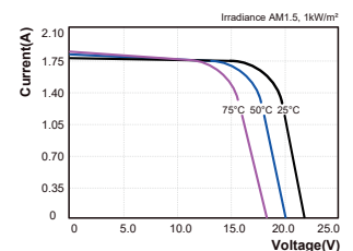
Curvas I-V del módulo PV ESF-20PC a varias temperaturas de celda I-V Curves of PV module ESF-20PC at various cell temperatures
