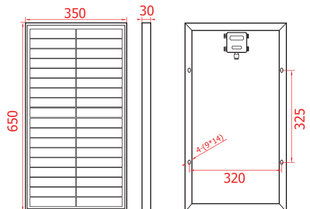
Dimensiones - Dimensions ESF-30PA
