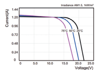
Resultado de la medición de potencia PVP Result of PVP Power Measurement
