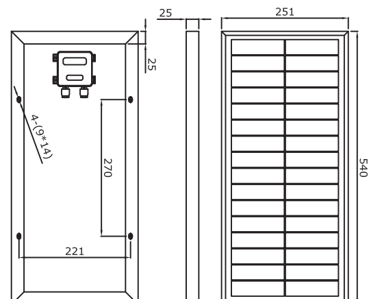
Dimensiones - Dimensions ESF-20MD
