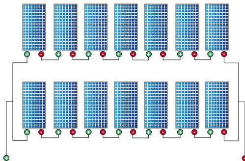
Installation pour pompe 220V 1. Connectez deux ensembles de sept panneaux 35V en parallèle. 2. Connectez les deux ensembles l'un à l'autre en série.
