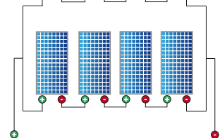
Instalación para bomba de 48V (Cuatro paneles de 17,5V conectados en serie)
