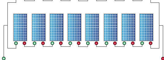
Instalación para bomba de 110V 1. Conectar dos conjuntos de ocho paneles de 17,5V en paralelo. 2. Conectar ambos conjuntos entre ellos en serie.
