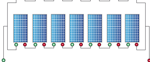
Instalación para bomba de 220V 1. Conectar dos conjuntos de siete paneles de 35V en paralelo. 2. Conectar ambos conjuntos entre ellos en serie.
