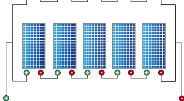
Instalación para bomba de 150V 1. Conectar dos conjuntos de cinco paneles de 30,5V en paralelo. 2. Conectar ambos conjuntos entre ellos en serie.
