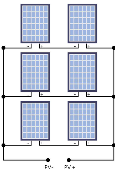
Paneles de 72 células en serie-paralelo en series de 2 unidades
