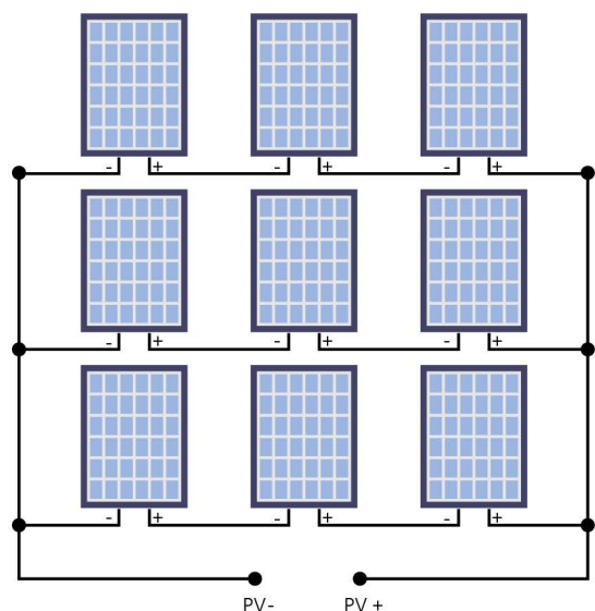
Paneles de 60 células en serie-paralelo en series de 3 unidades
