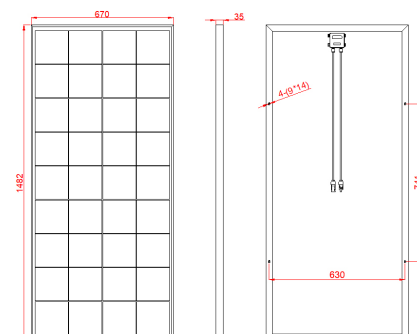
Dimensiones - Dimensions ESF-160PC
