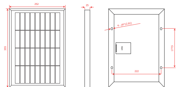
Dimensiones - Dimensions ESF-10PA
