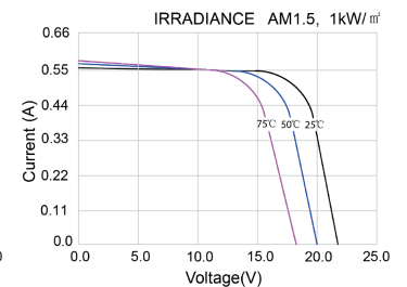
Curvas I-V del módulo PV ESF-10PA a varias temperaturas de celda I-V Curves of PV module ESF-10PA at various cell temperatures
